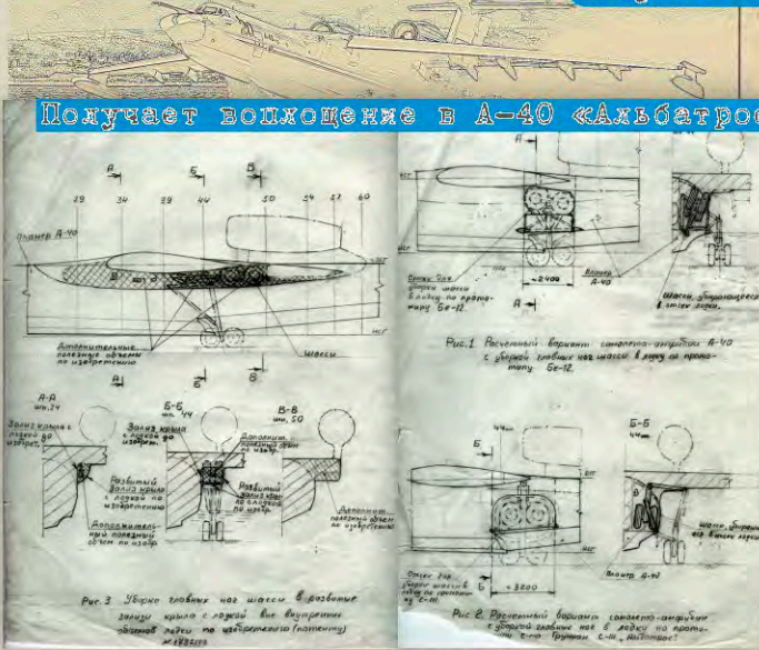
Предложение В. П. Гащенко по системе выпуска пиласы
